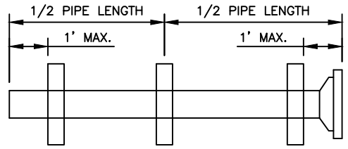
DI PIPE CASING SPACER DETAIL
