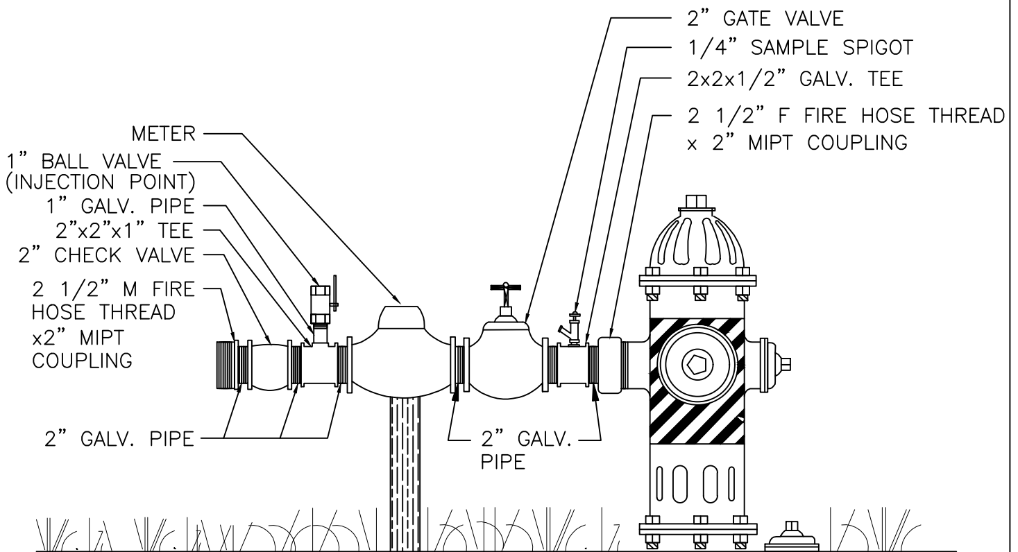
ELEVATION
